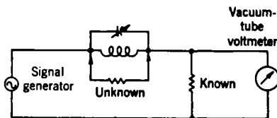
FIG. 2-18.—Voltage-divider circuit.
