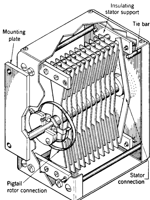
FIG. 9-17.—Bendix OAL-74747-1 sweep condenser.
