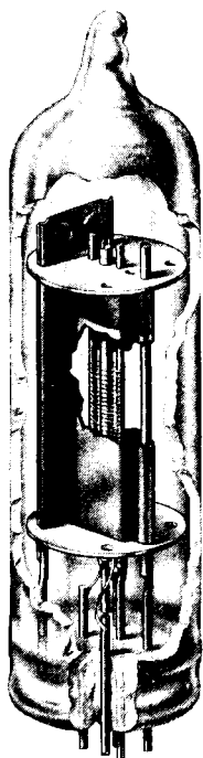
FIG. 14-10.—Subminiature triode 6K4.
