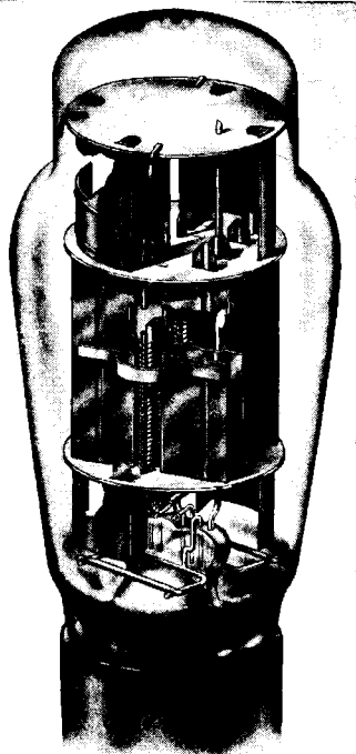
FIG. 14-9.—Twin low- \mu triode 6AS7G.
