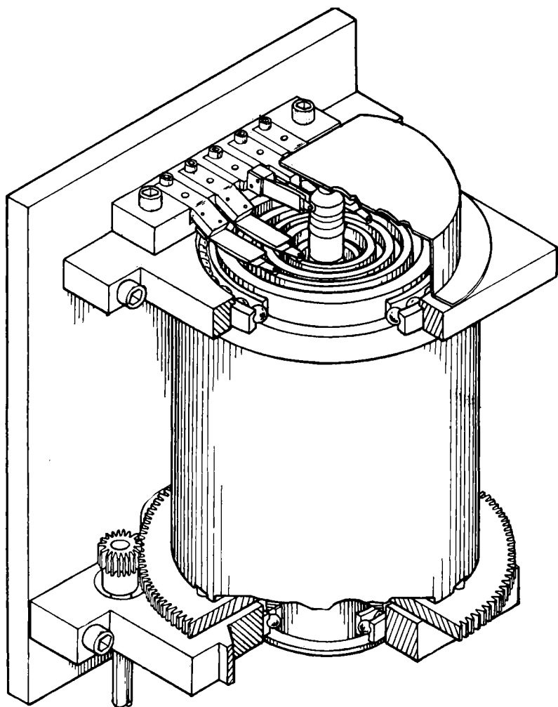
FIG. 10-9.—Synchro control motor.
