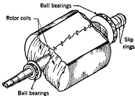
FIG. 10-5.—Synchro generator.
