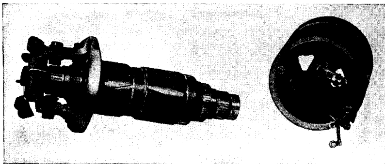
FIG. 12-6.—Bendix dynamotor.
